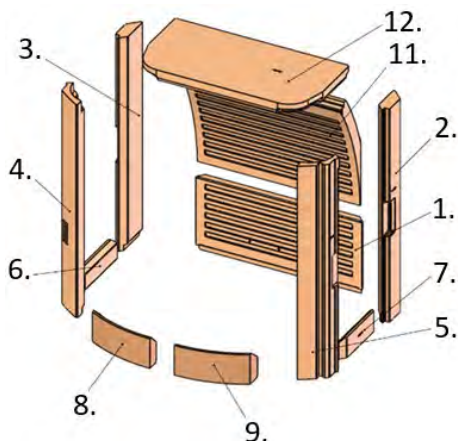
Figur 15 - Vermiculite samling
