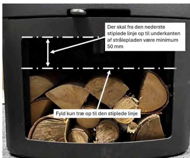
Figur 11 - Brænde opbevaring
